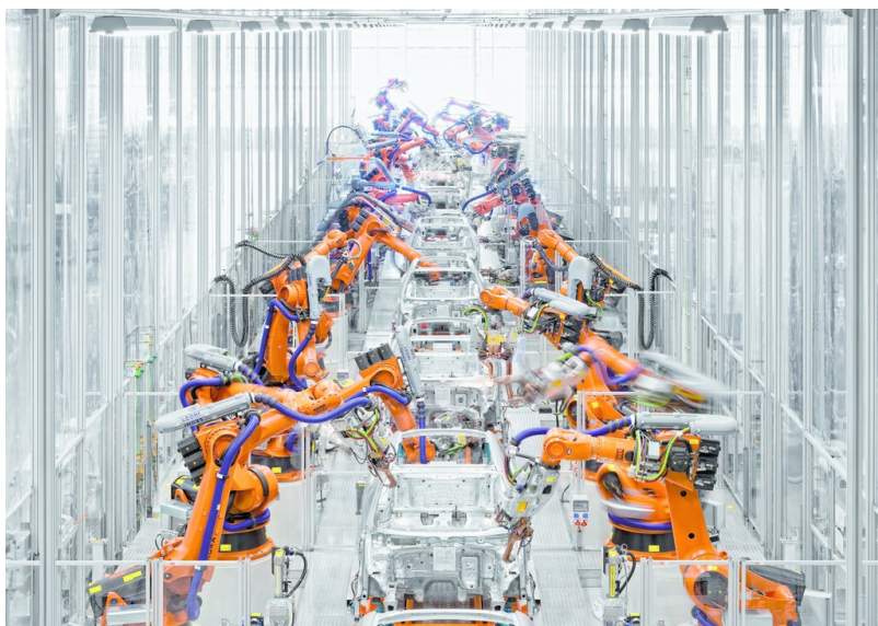
Karosseriebau im Audi-Werk Ingolstadt.
