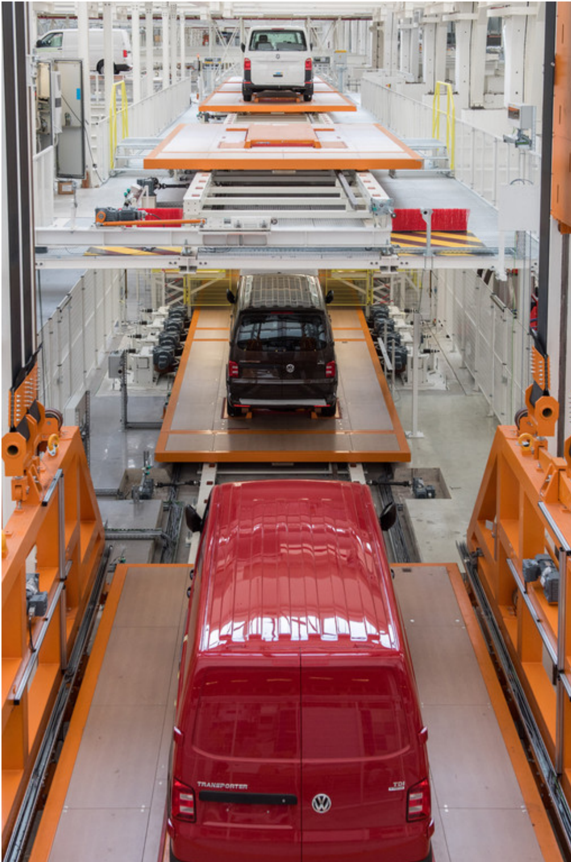
T6-Produktion im Volkswagen-Nutzfahrzeugwerk Hannover.
