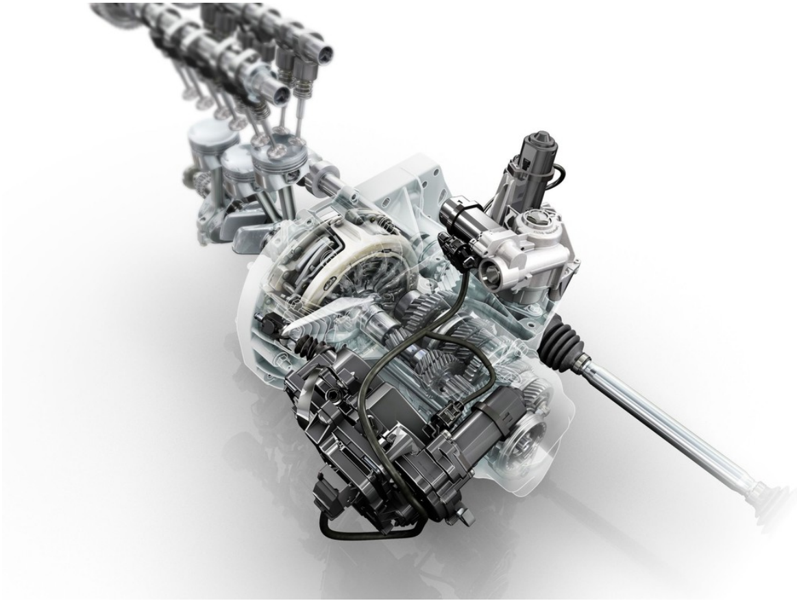
Automatisiertes Schaltgetriebe Easy-R von Dacia.
